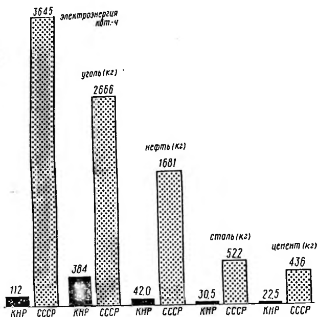
Производство важнейших видов промышленной продукции в КНР и СССР на душу населения
