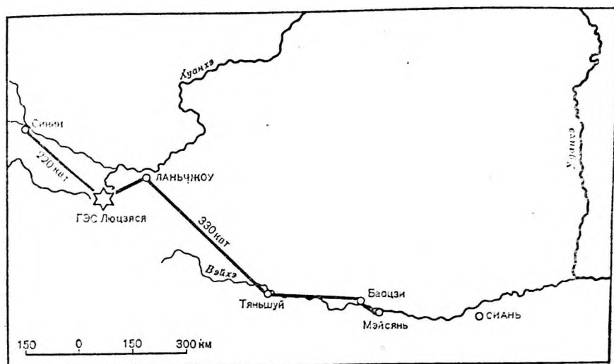
Схема 2. Высоковольтная линия электропередач Лютяньгуань
